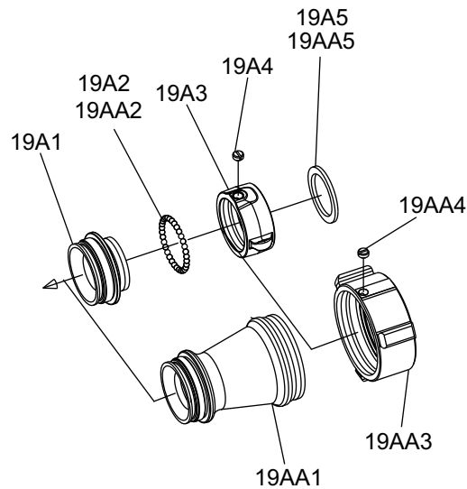
*1.5" OR 2.5" SWIVEL (STD)
